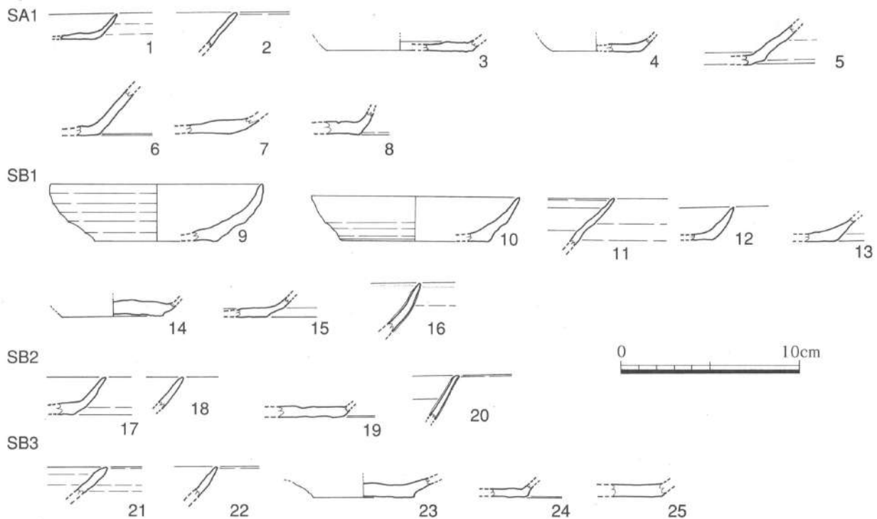
第4図 SA1・SB1～3出土遺物実測図(S=1/3)
