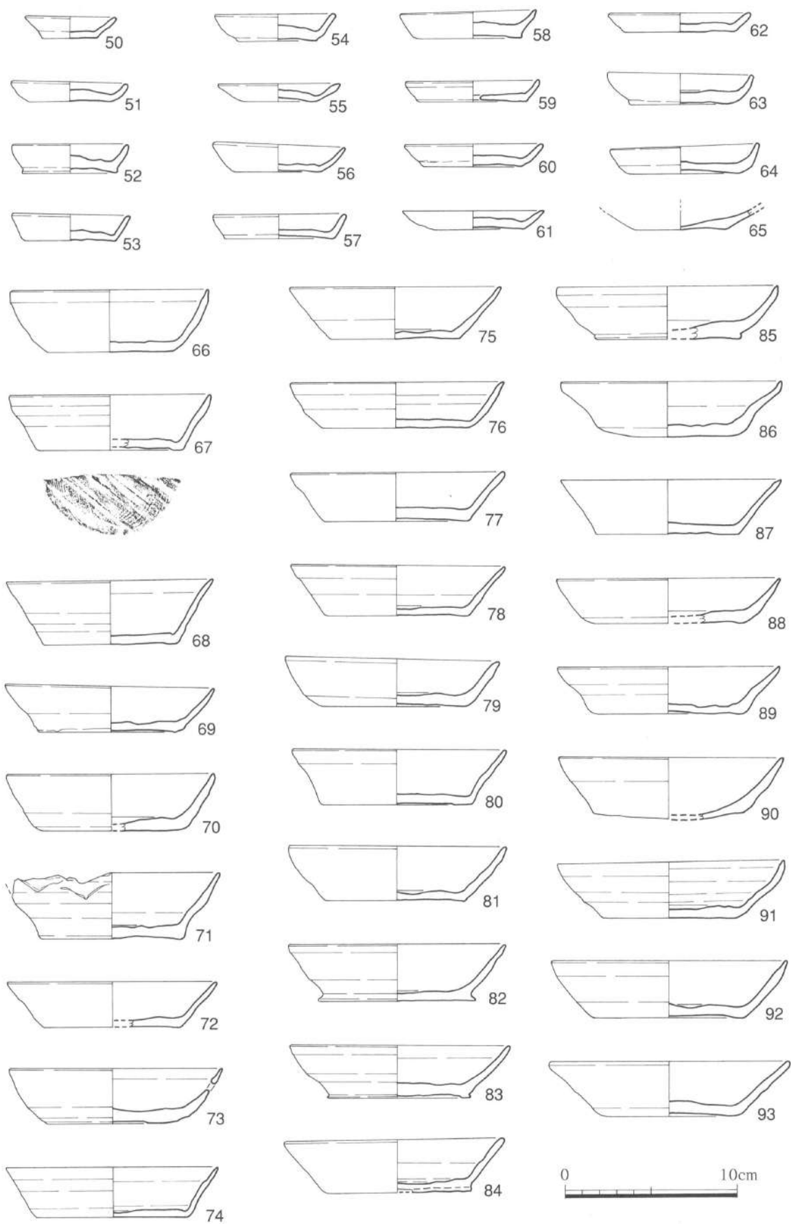
第14図 SE1出土遺物実測図1 (S=1/3)
