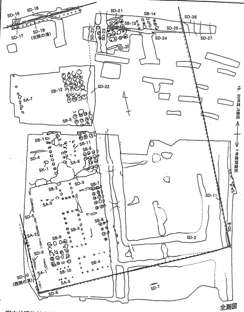
長者屋敷遺跡位置図・全測図・掘立柱建物跡実測図 (縮尺 1=1/3000、2=1/1000、他は 1/160)
