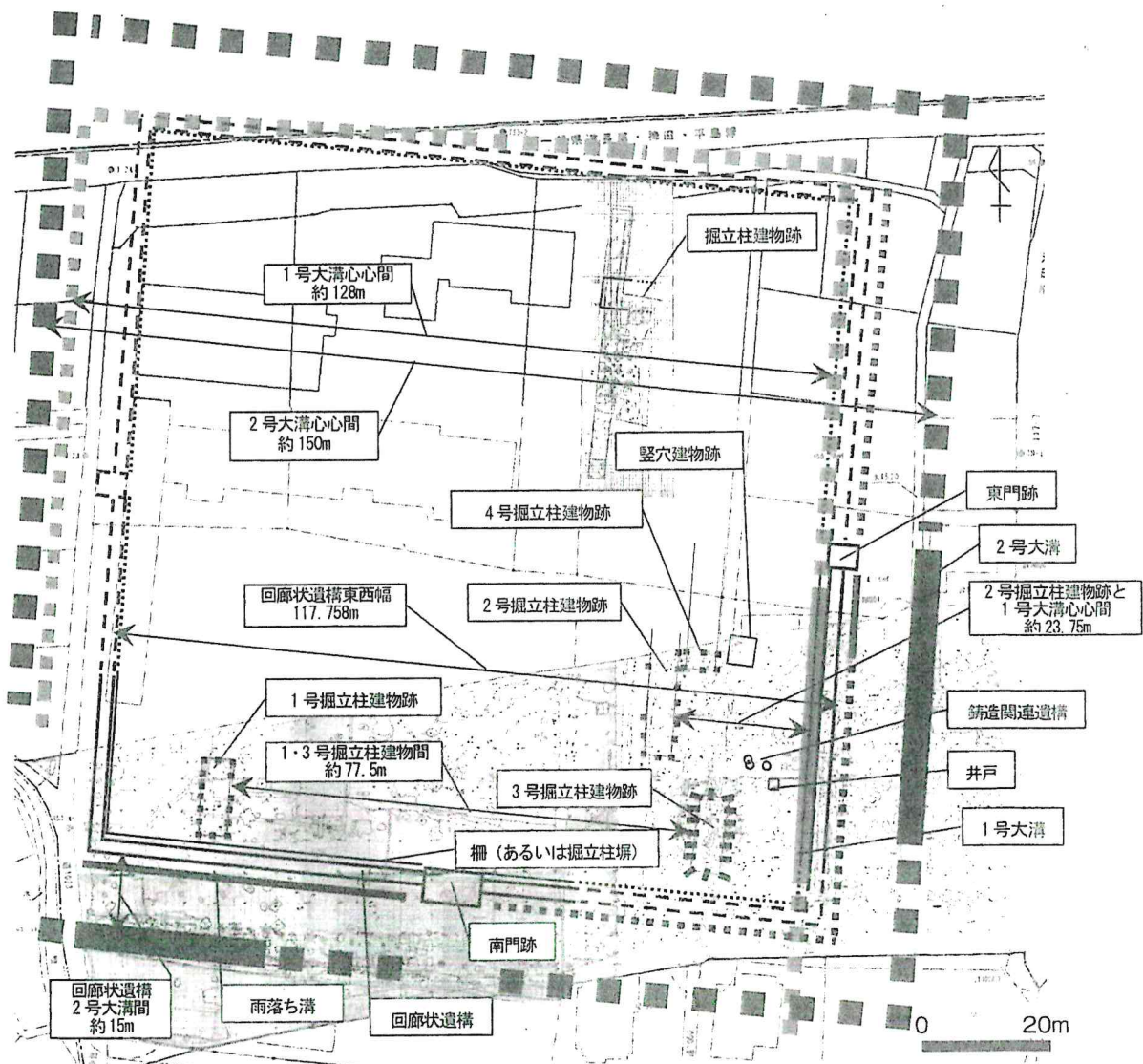
福原長者原遺跡政庁規模および遺構配置
