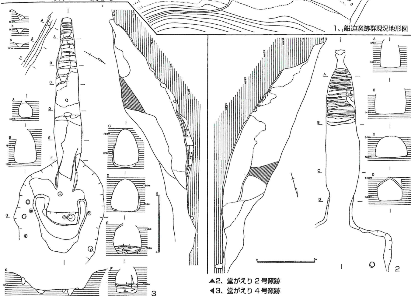
船迫窯跡群現況地形図及び窯跡実測図 (縮尺 1=1/200、2・3=1/120)
