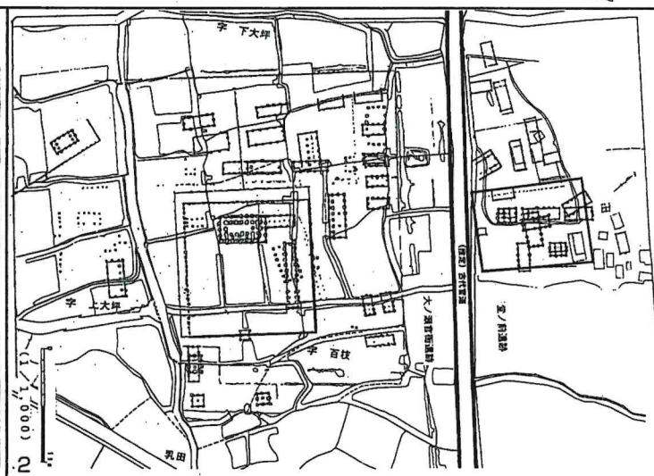
大ノ瀬官衙遺跡全測図及び出土遺物実測図 (縮尺 1=1/1200、2=1/3000、他は 1/6)
