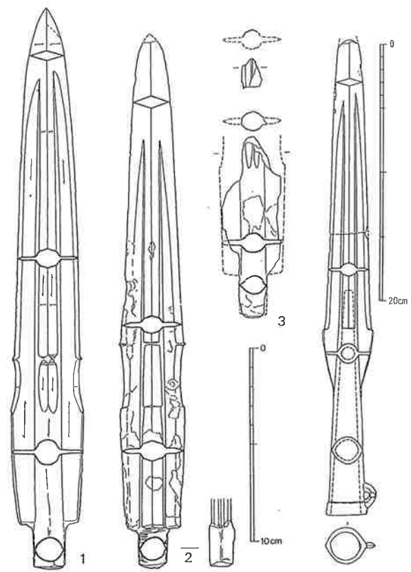
赤崎・吉井・向原出土の銅剣実測図
