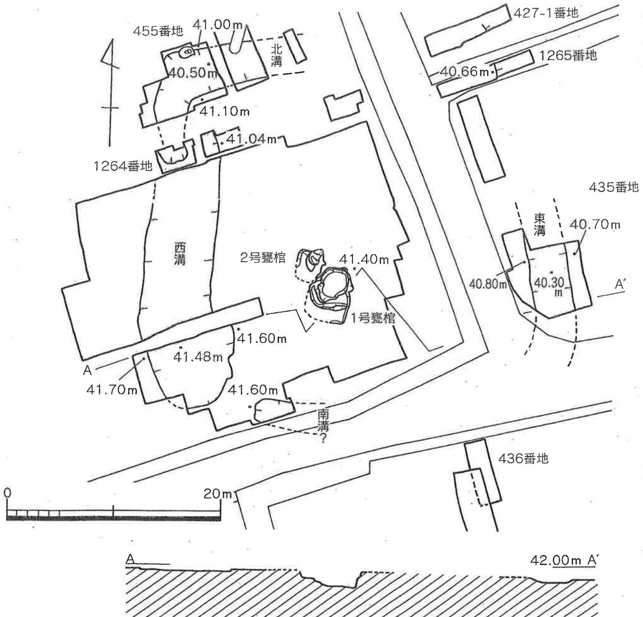
三雲南小路遺跡遺構配置と断面概略図 (1/400)
